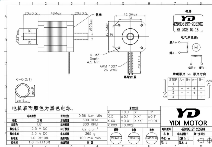
电机参数表 Motor parameter table
