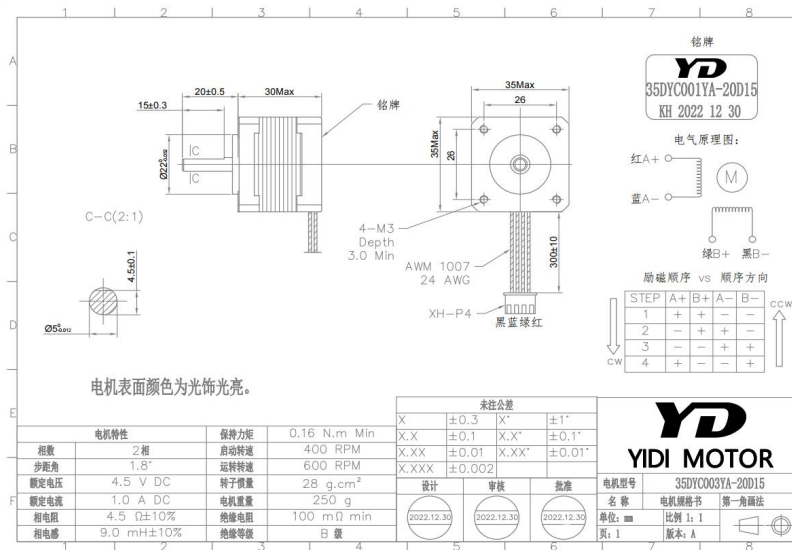
电机参数表 Motor parameter table
