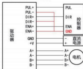
共阴极接法（高电平有效）
