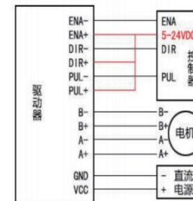
共阳极接法（低电平有效）
