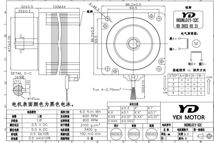
电机参数表 Motor parameter table
