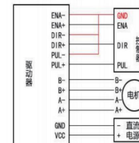
共阴极接法（高电平有效）
