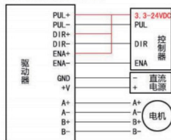
共阳极接法（低电平有效）
