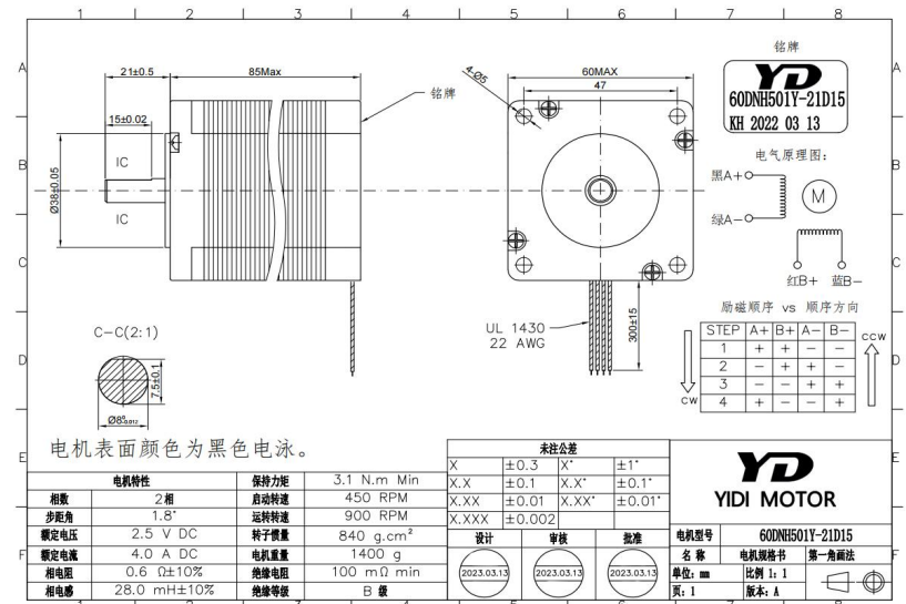
电机参数表 Motor parameter table
